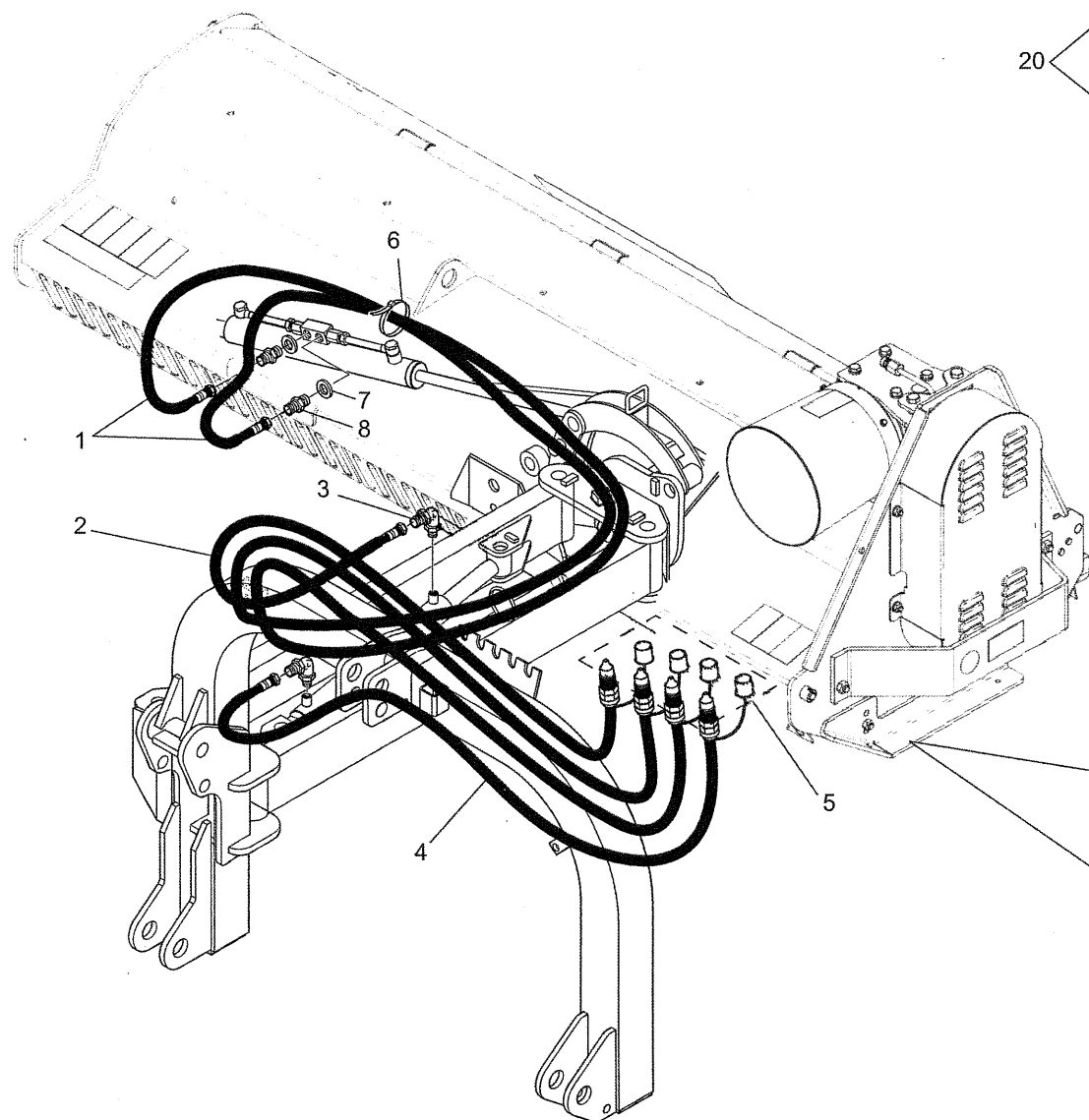
KIT RIDUZIONE TUBI IDRAULICI HYDRAULIC TUBE REDUCTION KIT
