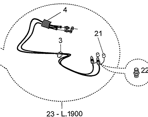
KIT RIDUZIONE TUBI IDRAULICI OPTIONAL OPTIONAL HYDRAULIC TUBE REDUCTION KIT
