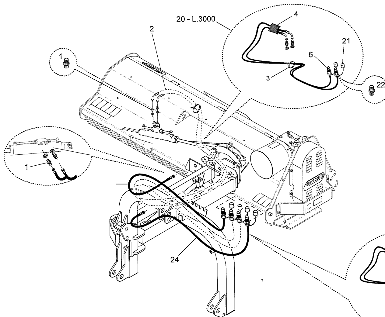
KIT RIDUZIONE TUBI IDRAULICI OPTIONAL OPTIONAL HYDRAULIC TUBE REDUCTION KIT
