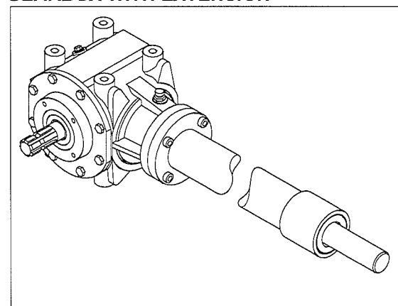
MOLTIPLICATORE CON PROLUNGA GEARBOX WITH EXTENSION
