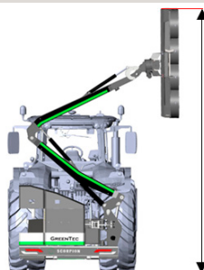
Räckvidd lodrätt
