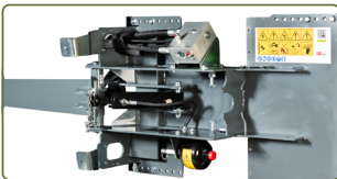
AHS hydraulisk påkörningssäkring med redskapsretur, detta optimerar arbetet och säkrar maskinen från överbelastning (standardutrustning).
