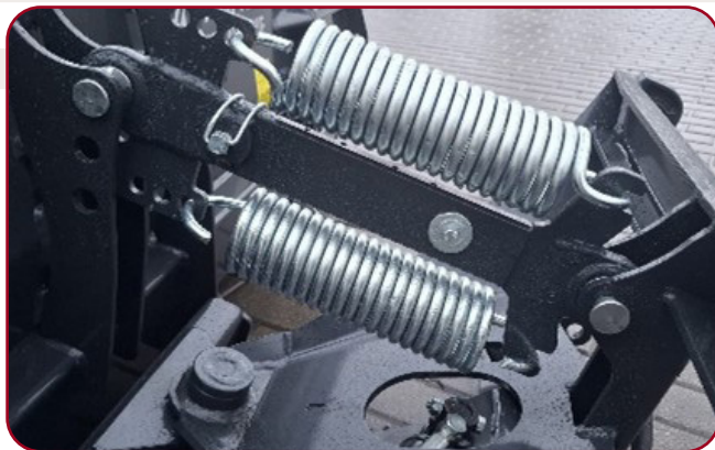
Fjäderutlösning
